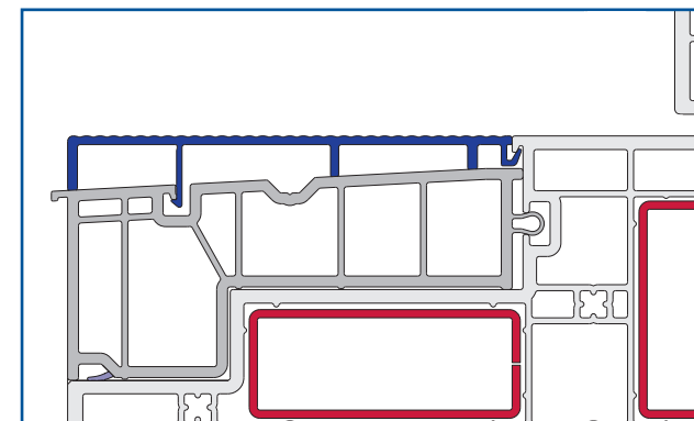
Barrierefreie Schwelle
