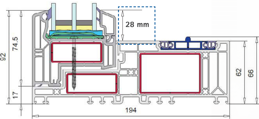
Innenansichtshöhe des Festflügels: 28 mm
